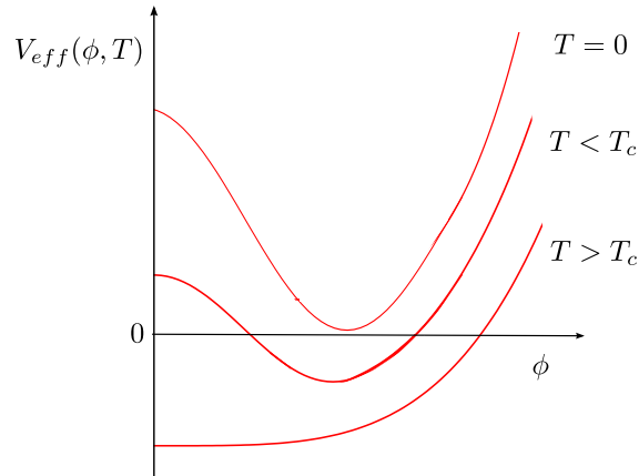
Figura 1.4: Potencial Efetivo
